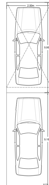
Planta Estacionamento - esc. 1|100
