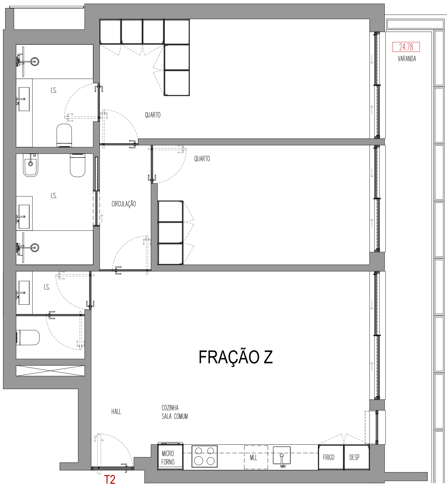
BLOCO D - FRAÇÃO Z - PISO 1
