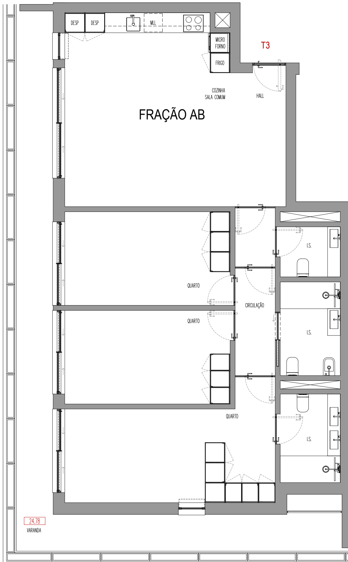
BLOCO D - FRAÇÃO AB - PISO 1
