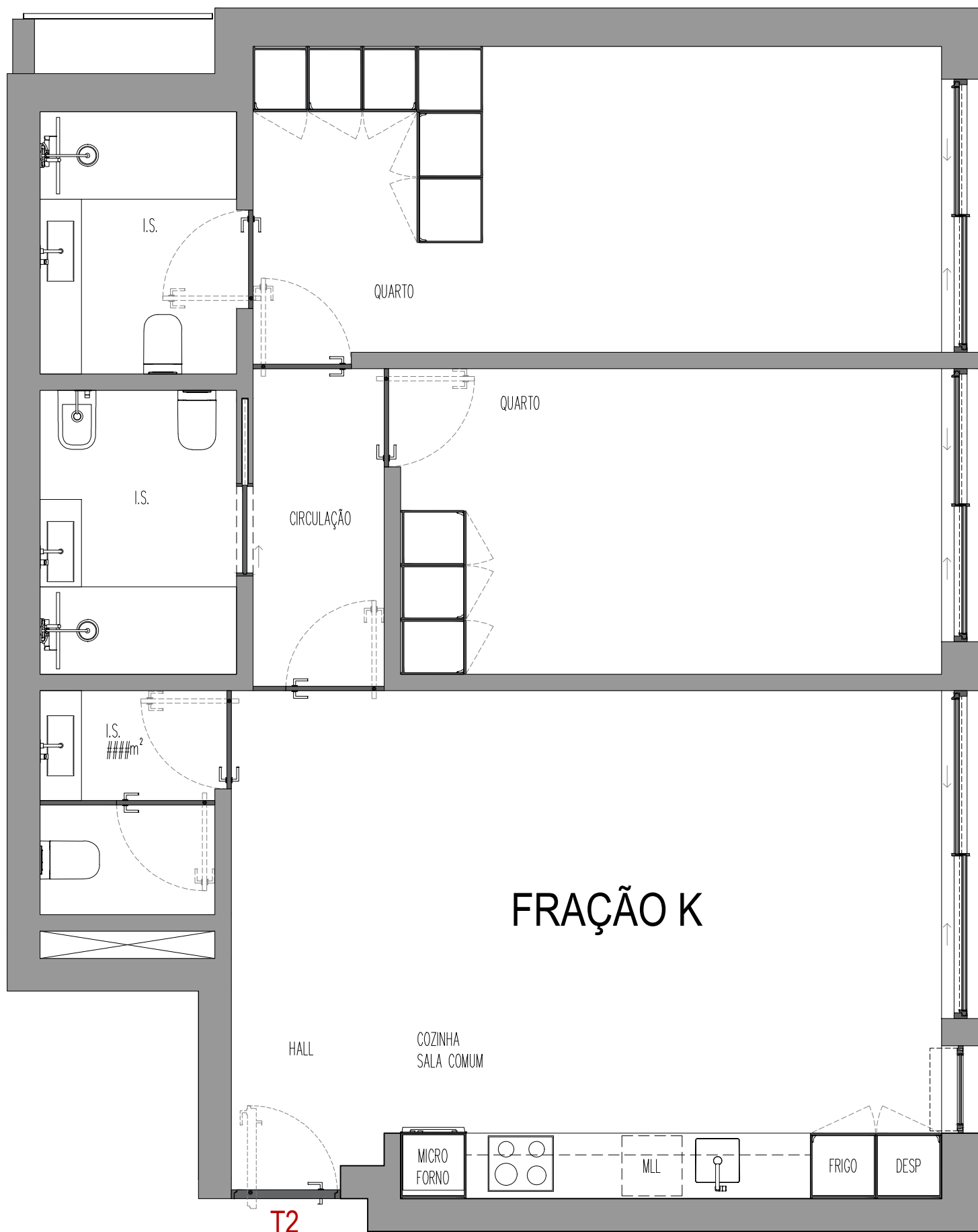
BLOCO D - FRAÇÃO K - PISO 0
