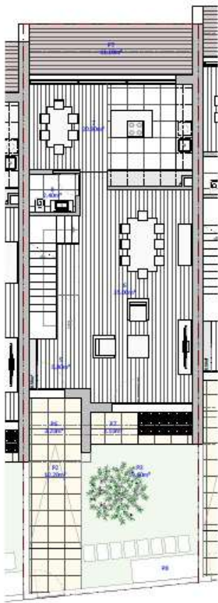
PLANTA DO PISO 1 escala 1/100
