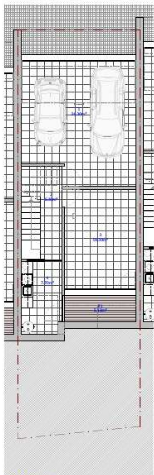
PLANTA DO PISO -1 escala: 1/50
