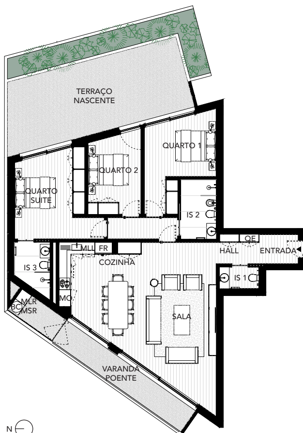
PLANTA PISO 1
